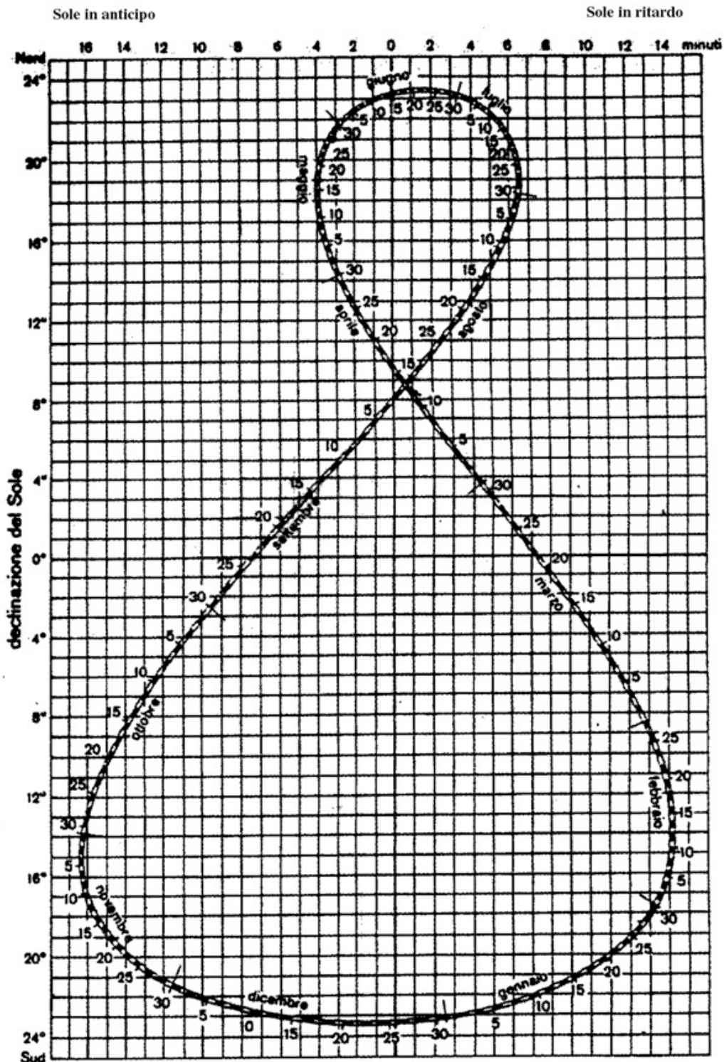
declinazione del Sole ed Equazione del tempo
